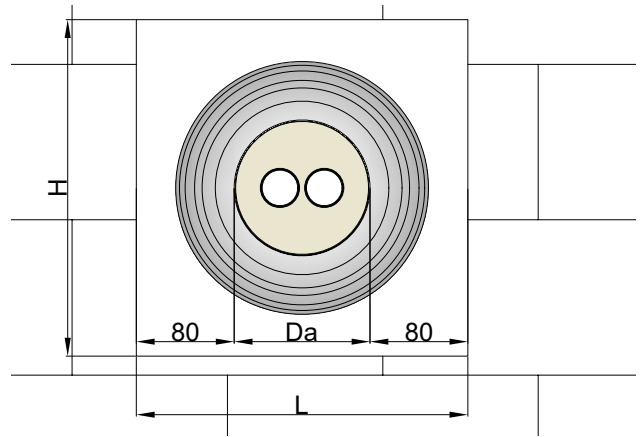
Abb. 37: Mauerdurchbruch FibreFLEX/CaldoPEX double
