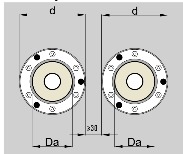
Abb. 43: Abstand zwischen 2 Kernbohrungen oder Futterrohren
