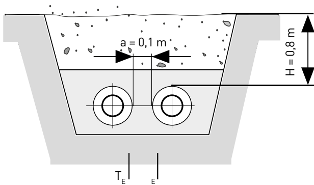
Abb. 24: Rohrgraben single-Rohr
