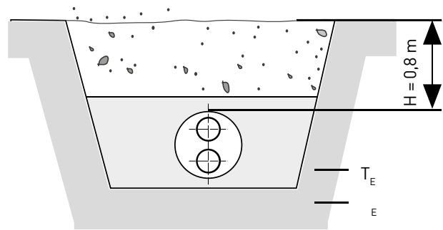
Abb. 25: Rohrgraben double-Rohr
