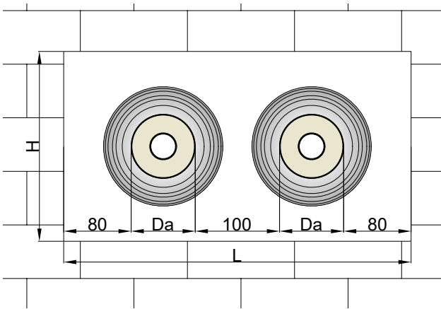
Abb. 36: Mauerdurchbruch FibreFLEX/CaldoPEX-Rohr single
