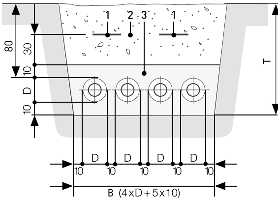
Abb. 33: Grabenquerschnitt 3 Rohre
