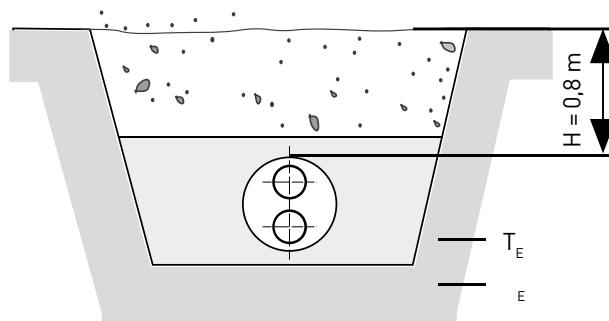
Abb. 21: Rohrgraben double-Rohr
