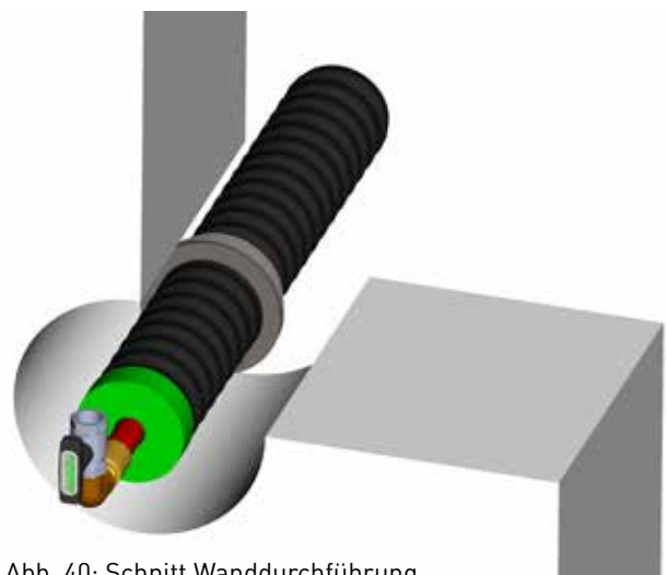
Abb. 40: Schnitt Wanddurchführung
