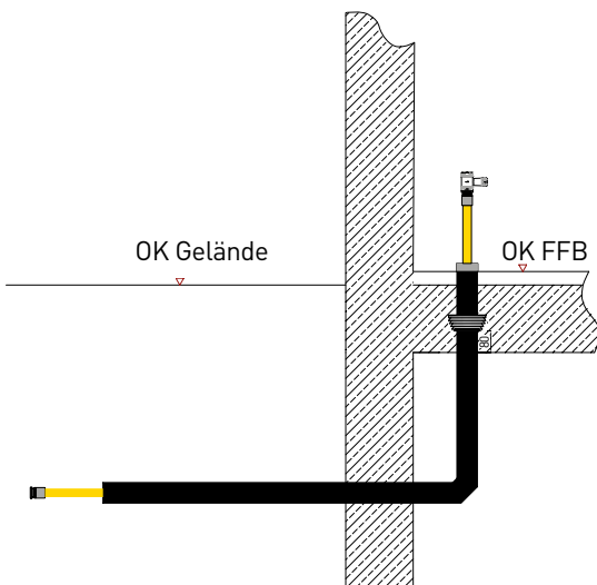
Abb. 52: Einbaubeispiel Hauseinführungsbogen
