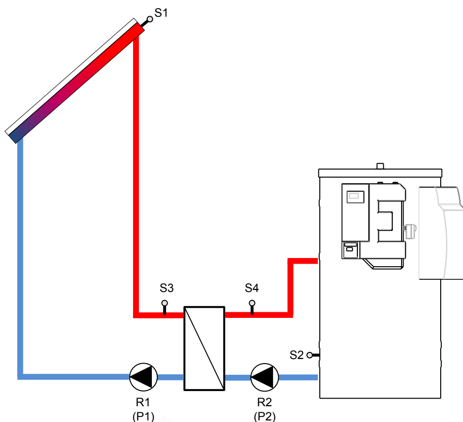
Abb. 63: Anschlussschema Solaranbindung
