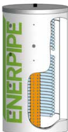
Abb. 53: Hygienepuffer
