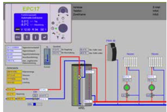
Abb. 39: Bildschirmanzeige Abnehmer
