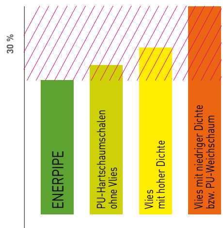
Abb. 7: Vergleich Dämmeigenschaften
