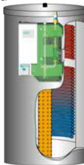
HPDL mit Ultraschall-Wärmemengenzähler
