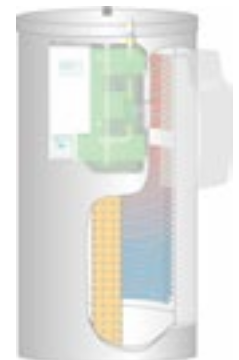
HPDL mit Frischwasserstation und Ultraschall-Wärmemengenzähler
