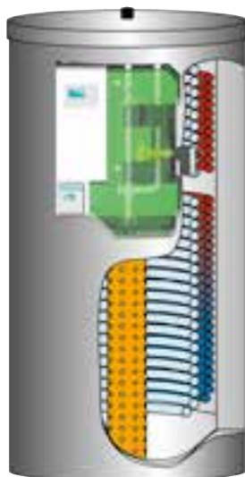
HPZL-H mit Ultraschall-Wärmemengenzähler
