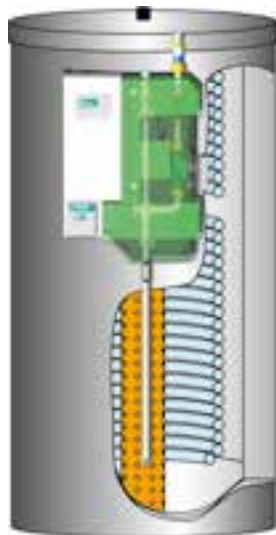
SPDL-H mit Ultraschall-Wärmemengenzähler
