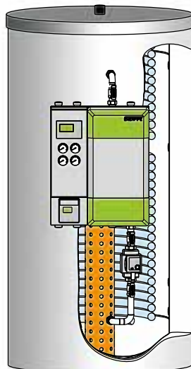
ÜSPZL-H mit Ultraschall-Wärmemengenzähler
